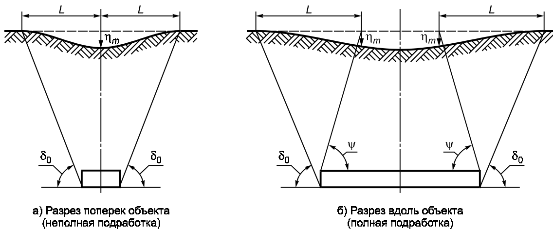
Рисунок С.1 — Основные параметры мульды сдвига
